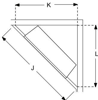
Dimensions pour installation en coin
