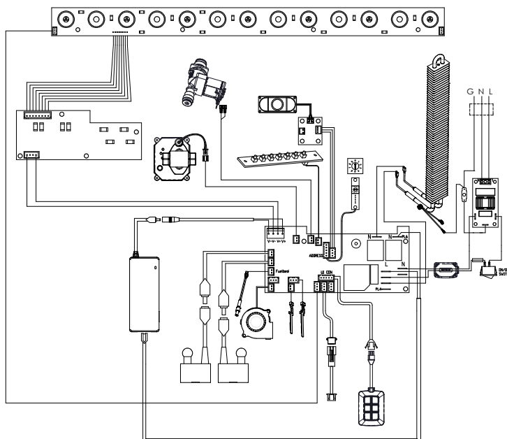
Schéma de câblage de la cassette
